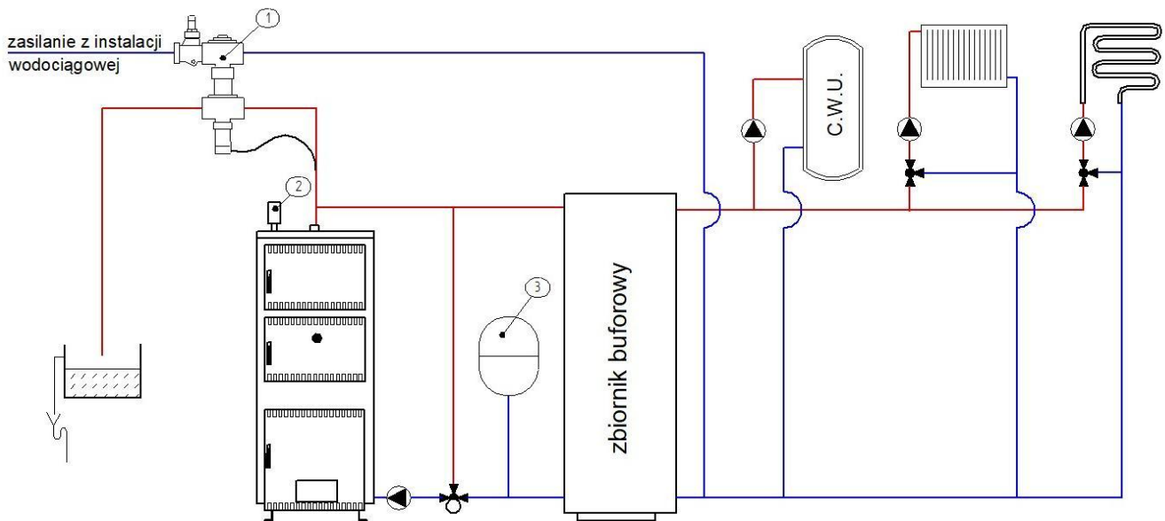
1- zabezpieczenie termiczne 5067 2 - zawór bezpieczeństwa 3 - przeponowe naczynie wzbiornice
